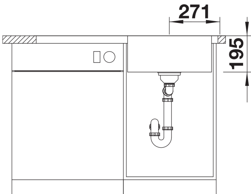
Frontansicht
